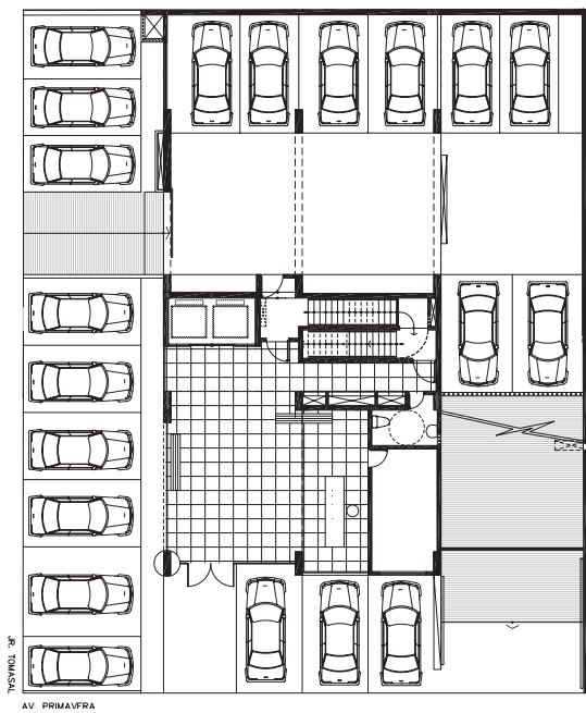
Planta típica
