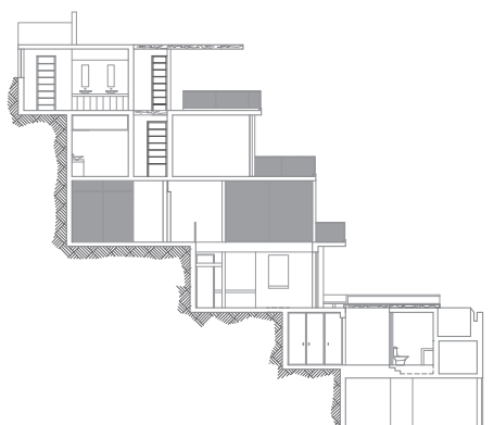
Corte
