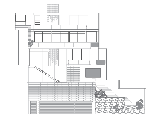
Elevación
