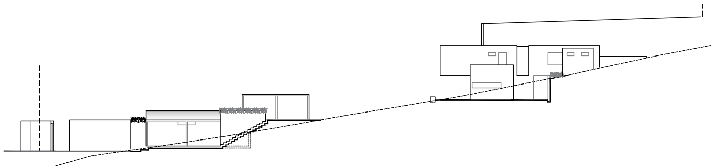
Elevación
