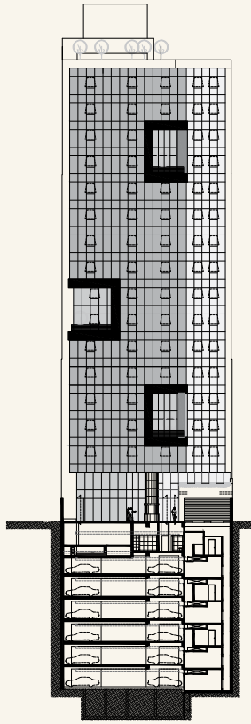
Corte - elevación frontal
