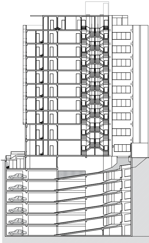
Corte
