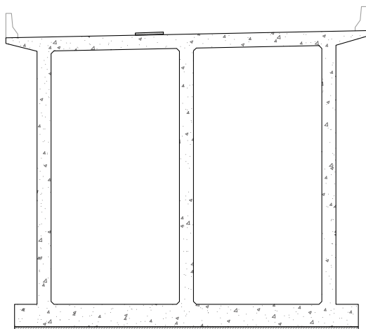
Detalle - Muro tipo marco
