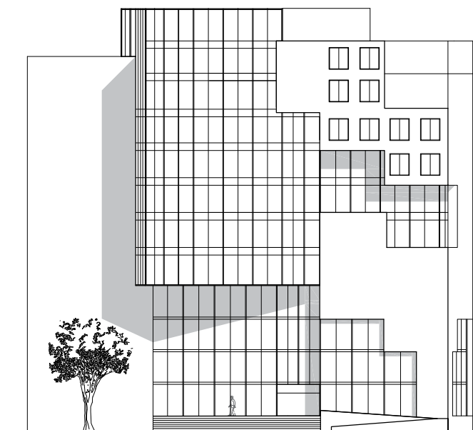
Elevación
