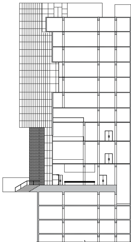
Corte
