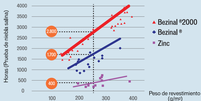
RESISTENCIA A LA CORROSIÓN ZINC PESADO - BEZINAL® - BEZINAL®2000
