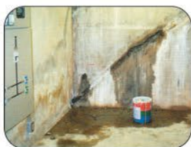
Etap 2 Reparación de Estructura con Radmyx
