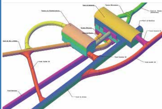
Gráfico N° 4: Túneles
